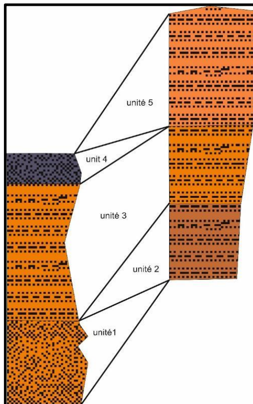
Figure 5 . Corrélation lithostratigraphique des puits 1 et 2
