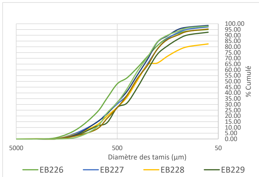
Figure 8. Courbe cumulative de type sigmoïde des sables du puits 2
