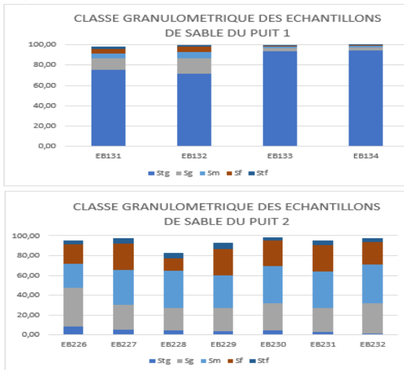
Figure 6. Classe granulométrique des sables des puits 1 et
