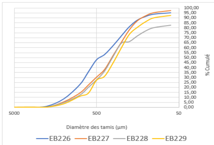
Figure 7. Courbe cumulative de type sigmoïde des sables du puits 1
