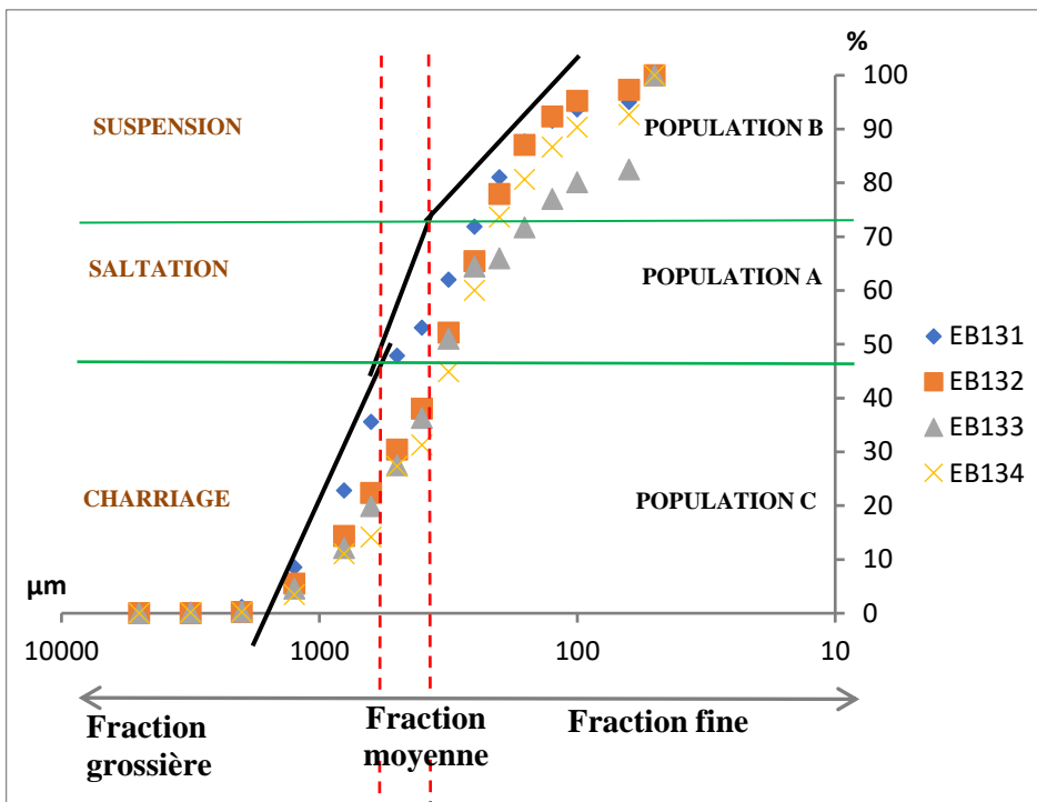
Figure 9. Diagramme de Visher (1969) appliqué aux sédiments du puits 1
