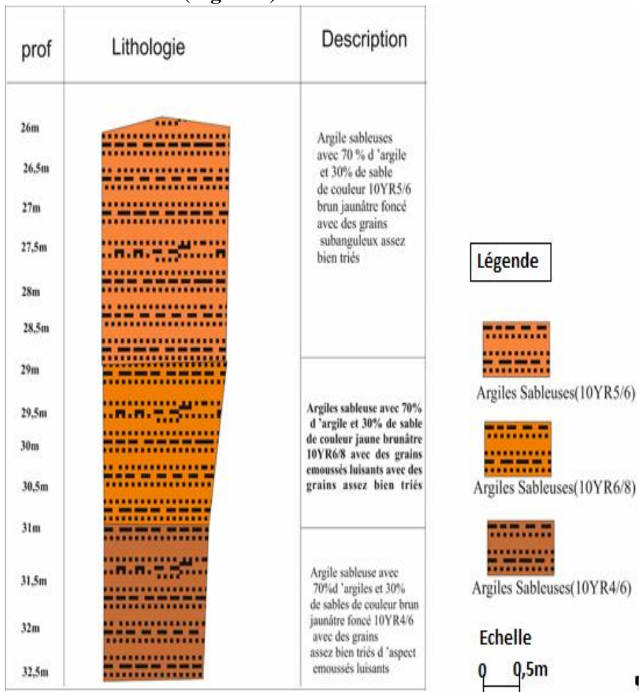
Figure 4. Coupe lithostratigraphique du Puits 2
