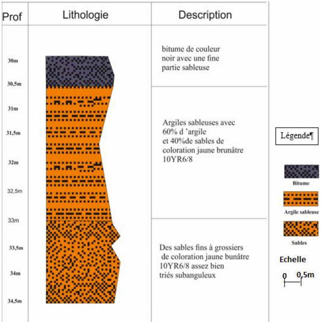
Figure 3. Coupe lithostratigraphique du Puits 1
