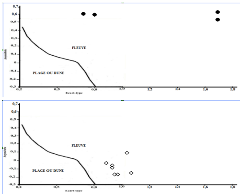
Figure 11 . Diagramme Sk-So de Friedman appliquée aux sédiments des puits 1 et 2
