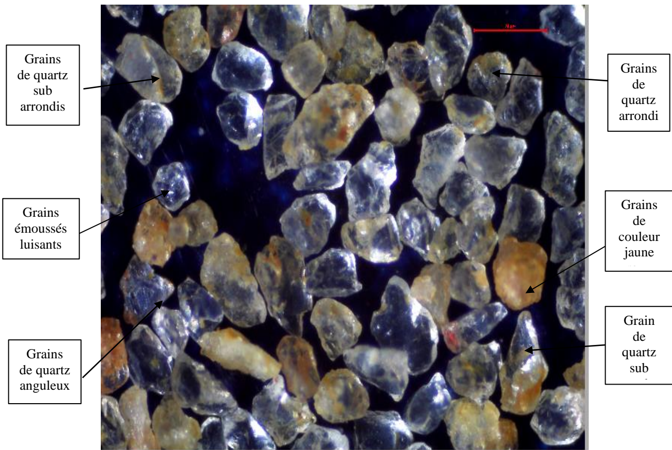
Figure 12. Morphoscopie des grains de sable de quartz (Forme et aspect des grains)
