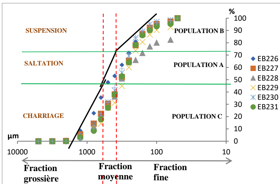
Figure 10. Diagramme de Visher (1969) appliqué aux sédiments du puits 2
