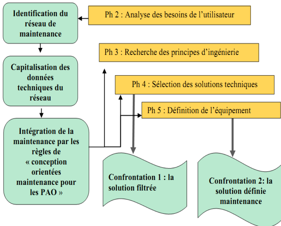
Fig.3 Démarche de Conception Orientée Maintenance (Bationo, 2007)
