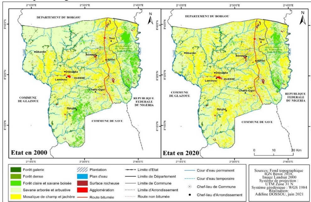
Figure 2. Occupation des terres entre 2000 et 2020 de la commune de Ouèssè
