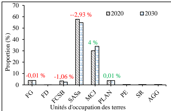
Figure 8. Evolution des unités d'occupation des terres de la commune de Ouèssè entre 2020 et 2030
