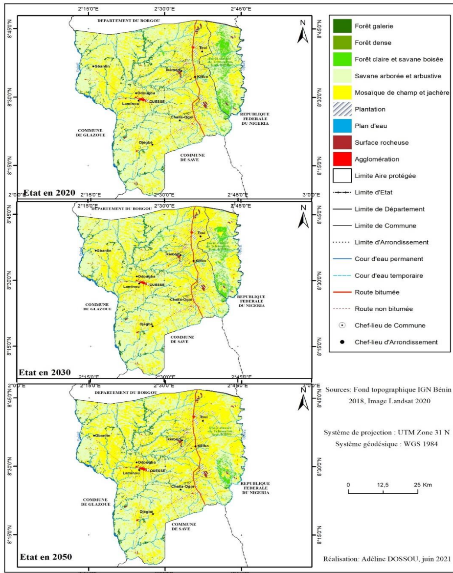
Figure 7. Prédiction de l'occupation des terres de la commune de Ouèssè à l'horizon 2030 et 2050
