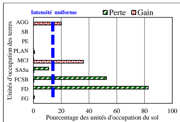
Figure 4. Intensité et vitesse des changements à l’intérieur de chaque catégorie d’occupation des terres entre 2000 et 2020
