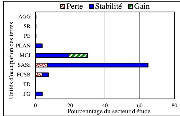
Figure 3. Intensité des changements par catégorie d’occupation des terres entre 2000 et 2020
