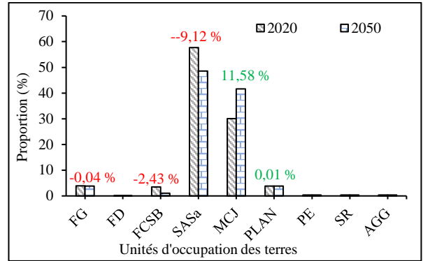
Figure 9. Evolution des unités d'occupation des terres de la commune de Ouèssè entre 2020 et 2050
