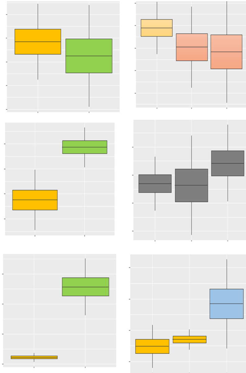
Figure 2 : Moyenne de la richesse, de l'abondance et de la densité du zooplancton (avec 95% d'intervalle de confiance)
