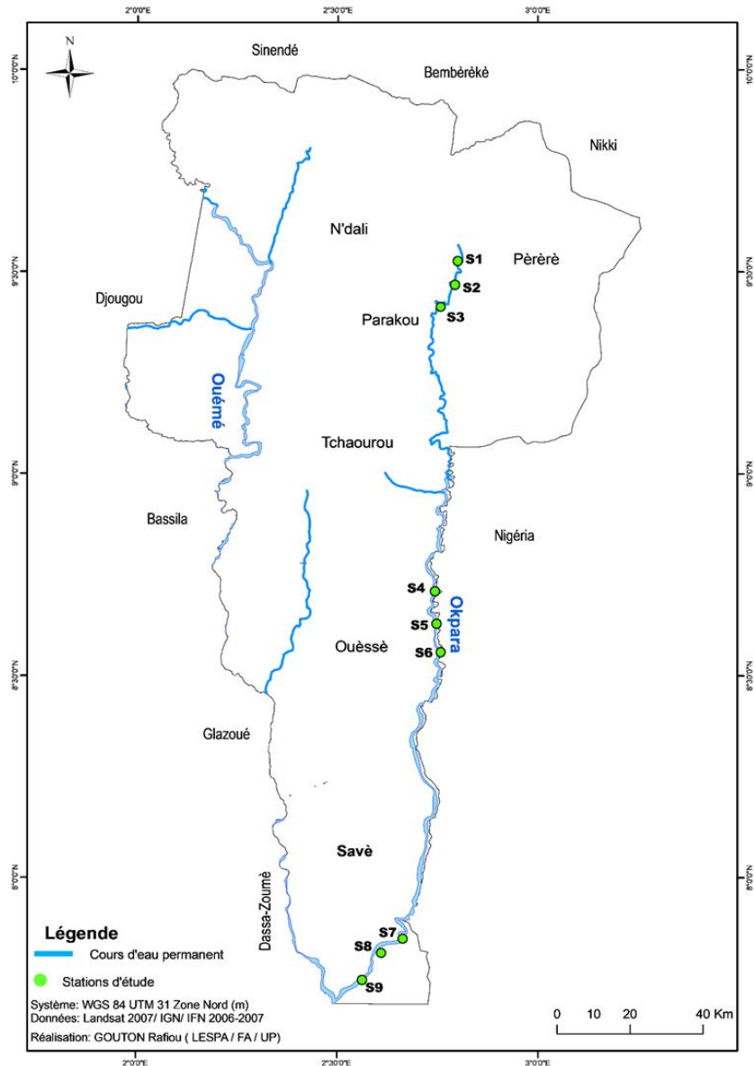
Figure 1 : Localisation de la rivière Okpara avec les stations d'étude
