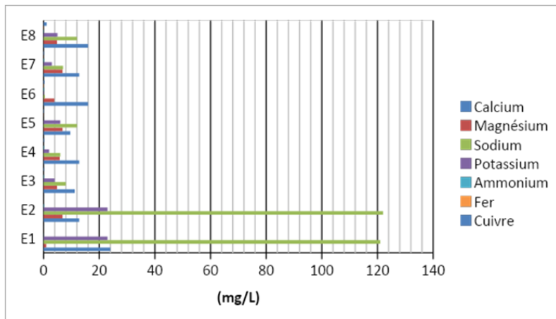
Figure 20: Teneurs en cations de Ca, K, Na, Mg Ca, Fe, Cu et d'Ammonium des eaux de surface à Tamourt En aj
