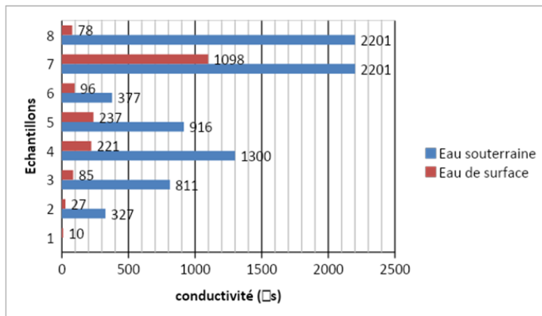
Figure 7: conductivité des eaux à Tamourt Naaj
