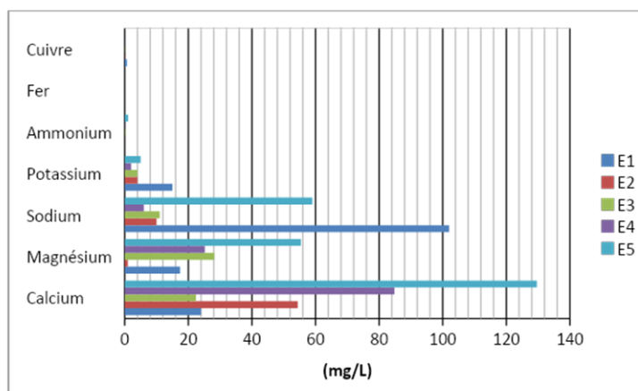
Figure 19 : Teneurs en cations de Ca, K, Na, Mg Ca, Fe, Cu et d'Ammonium des eaux souterraines à Mahmouda
