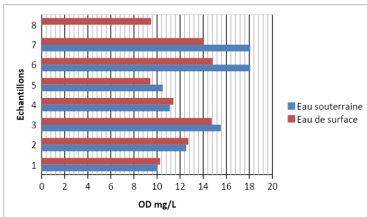
Figure 13 : La teneur en oxygène dissous des eaux de surface et souterraine à Tamourt En aj
