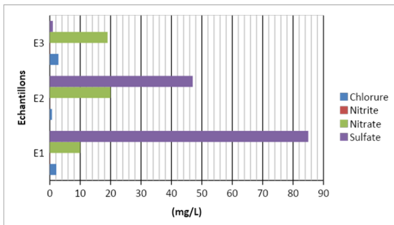
Figure 22: Teneurs en anions de Cl, Nitrite, Nitrate, \text{So}_4 des eaux de surface à Mahmouda
