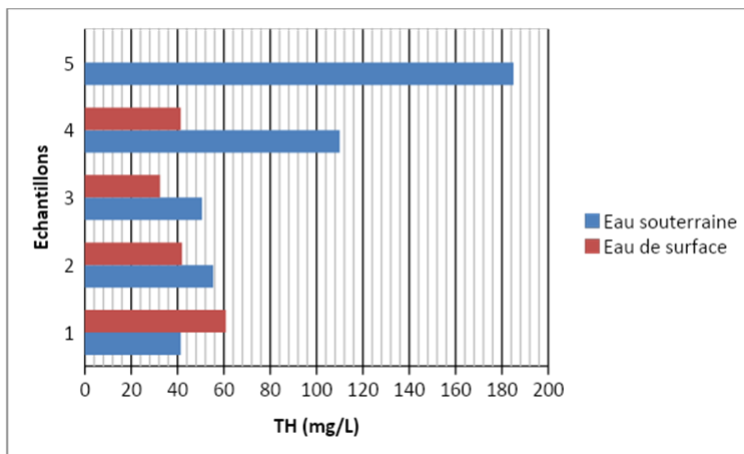
Figure 16: Dureté des eaux de surface et souterraine à Mahmouda
