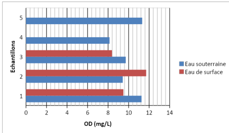
Figure 12: La teneur en oxygène dissous des eaux de surface et souterraine à Mahmouda
