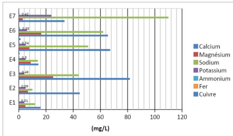
Figure 21 : Teneurs en cations de Ca, K, Na, Mg Ca, Fe, Cu et d'Ammonium des eaux souterraines à Tamourt En aj
