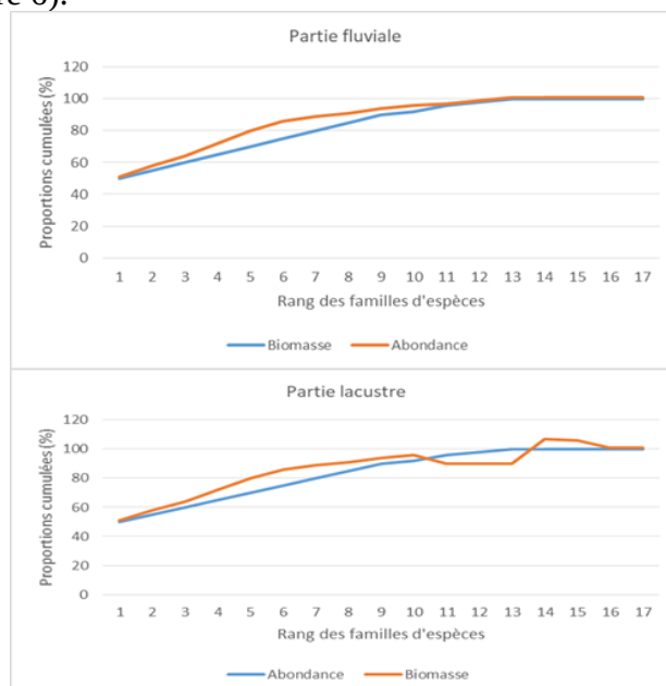
Figure 6 : Courbe ABC de la communauté de poissons des sites prospectés dans le bassin inférieur du fleuve Sassandra
