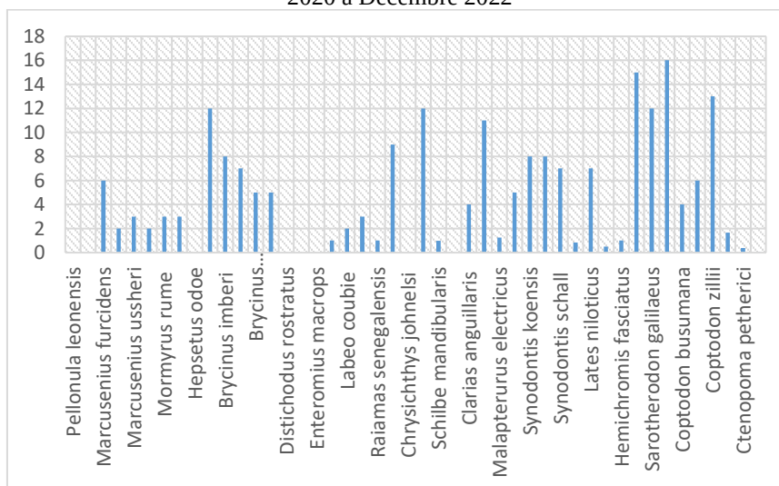
Figure 5 : Variation du nombre d'individus par espèce dans la partie fluviale à Buyo Juin 2020-Décembre 2022
