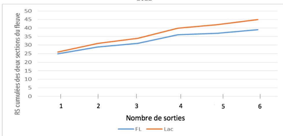
Figure 2 : Evolution des courbes de la richesse spécifique (RS) en fonction du nombre de jours de pêche cumulé sur les deux sections du fleuve Sassandra de juin 2020 à décembre 2022
