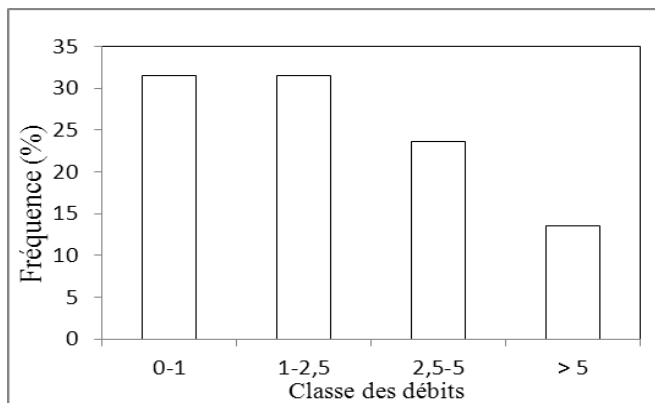
Figure 4: Histogramme des classes de débits de la région (CIEH, 1978)
