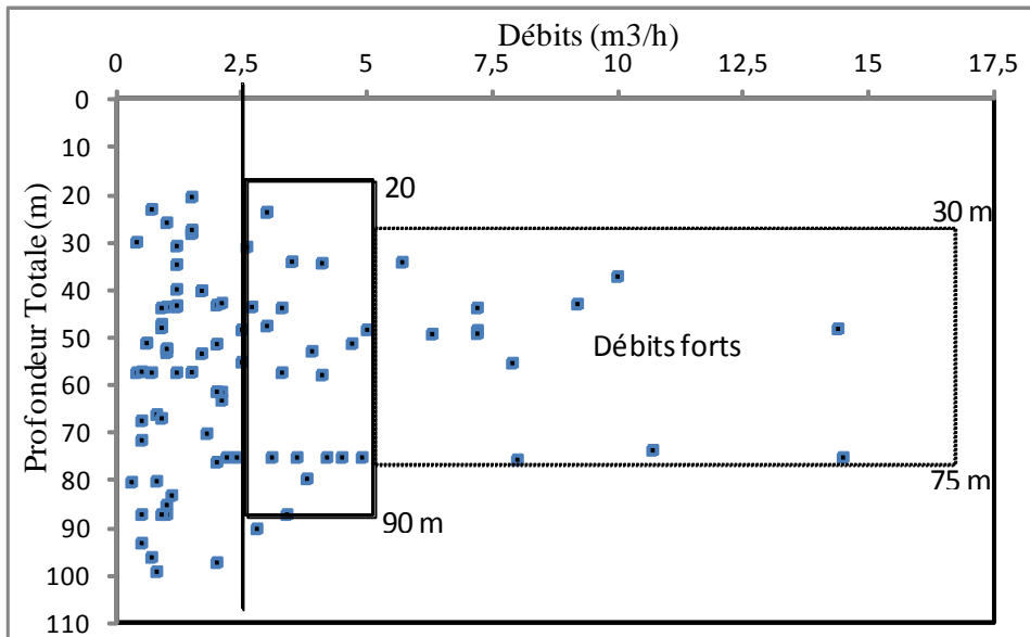
Figure 5 : Relation entre débits et profondeur totale des forages
