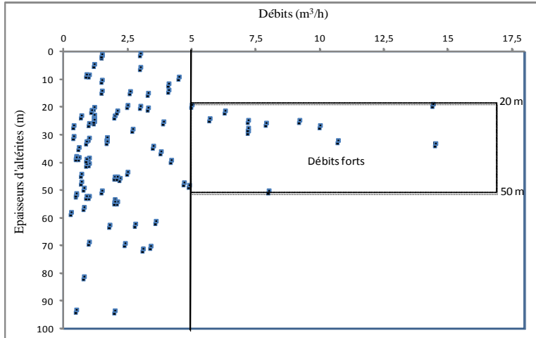
Figure 6 : Relation entre débits et épaisseur d’altérites
