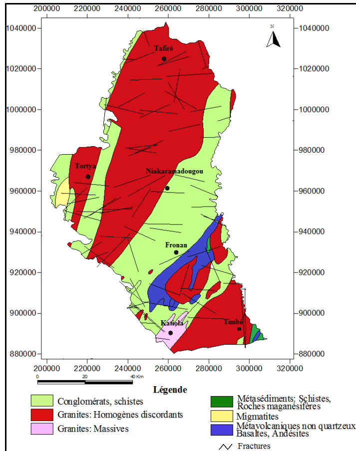
Figure 2 : Carte géologique de la région de Katiola
