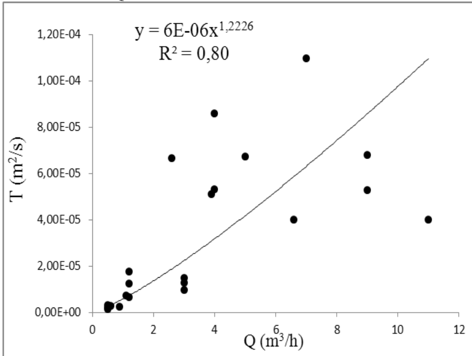
Figure 8 : Relation entre la transmissivité et le débit des forages
