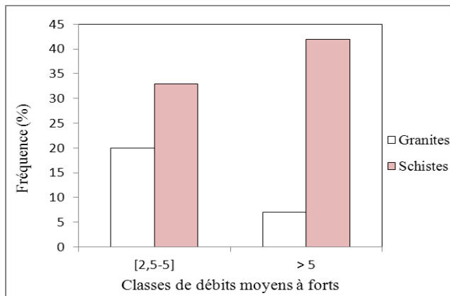
Figure 7: Productivité des ouvrages en fonction du type de formation
