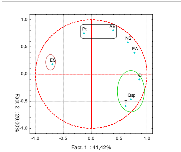
Figure 9: Projection des variables dans le plan F1-F2
