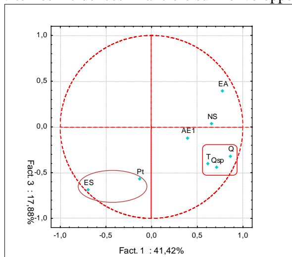
Figure 10: Projection des variables dans le plan factoriel F1-F3
