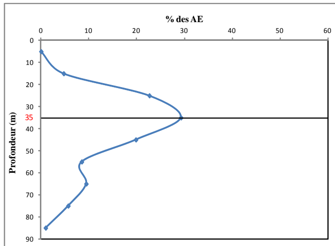
Figure 3: Relation entre AE et profondeur des forages dans le socle
