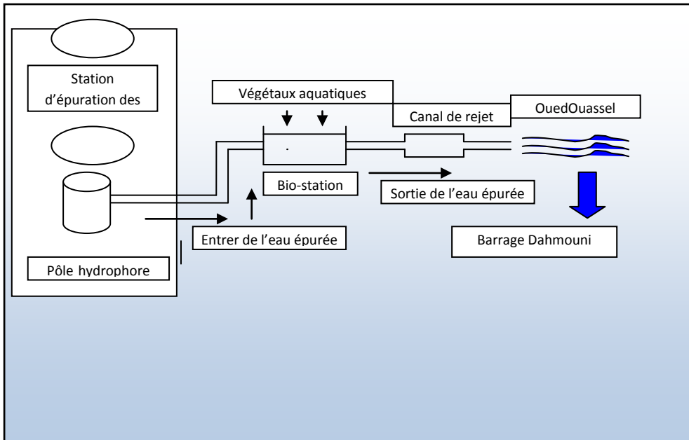
Figure .4. Schéma représentatif de l'implantation de la bio-station dans la station d'épuration de Tiaret.
