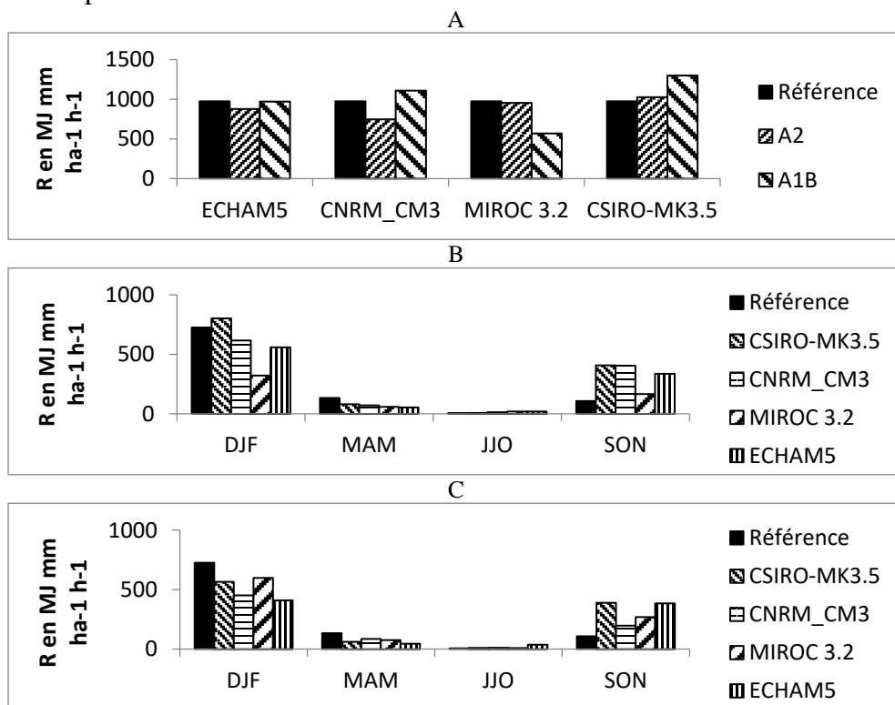
Figure 6 : Tendances futures du facteur R par rapport à la référence. A : annuelles, B : saisonnières selon le scénario A1B, C : saisonnières selon le scénario A2.
